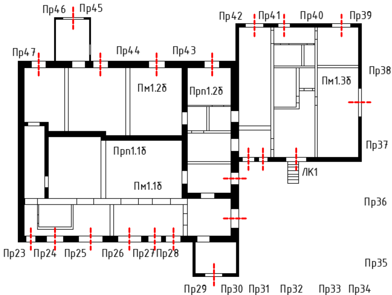
Б-План 2-ого этажа
