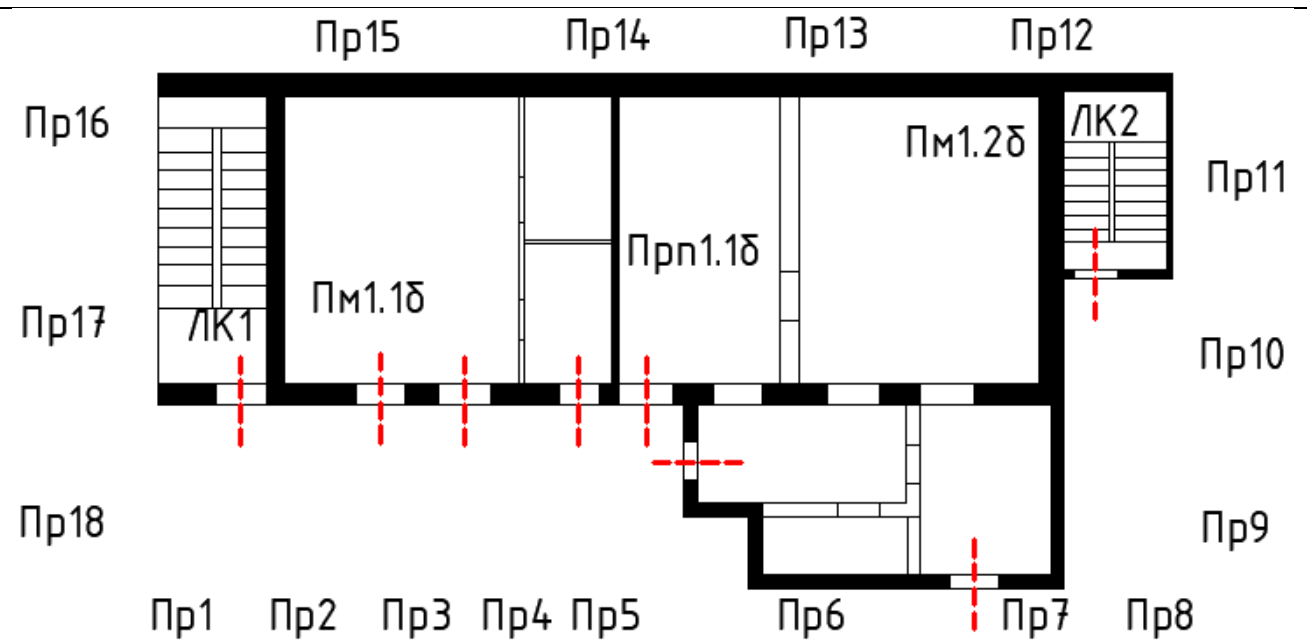
Б-План 1-ого этажа
