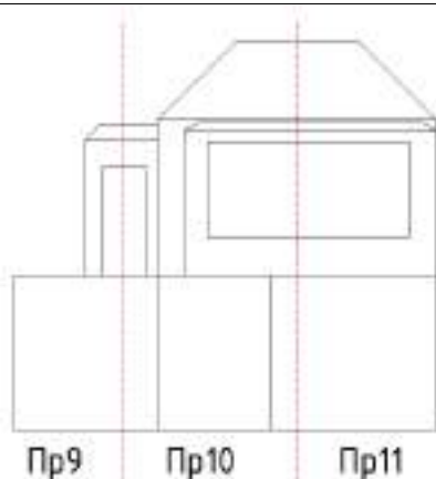
Б-Фасад 3 (фундамент 3, стена 3, покрытие 3)
