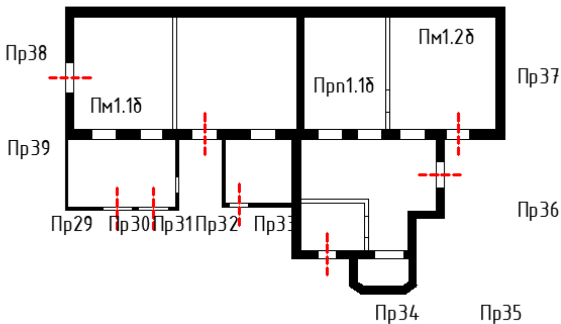
Б-Фасад 1 (фундамент 1, стена 1, покрытие 1)
