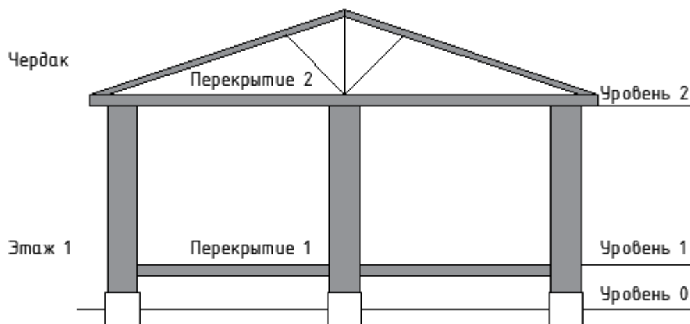
А,Б-Схема разреза
