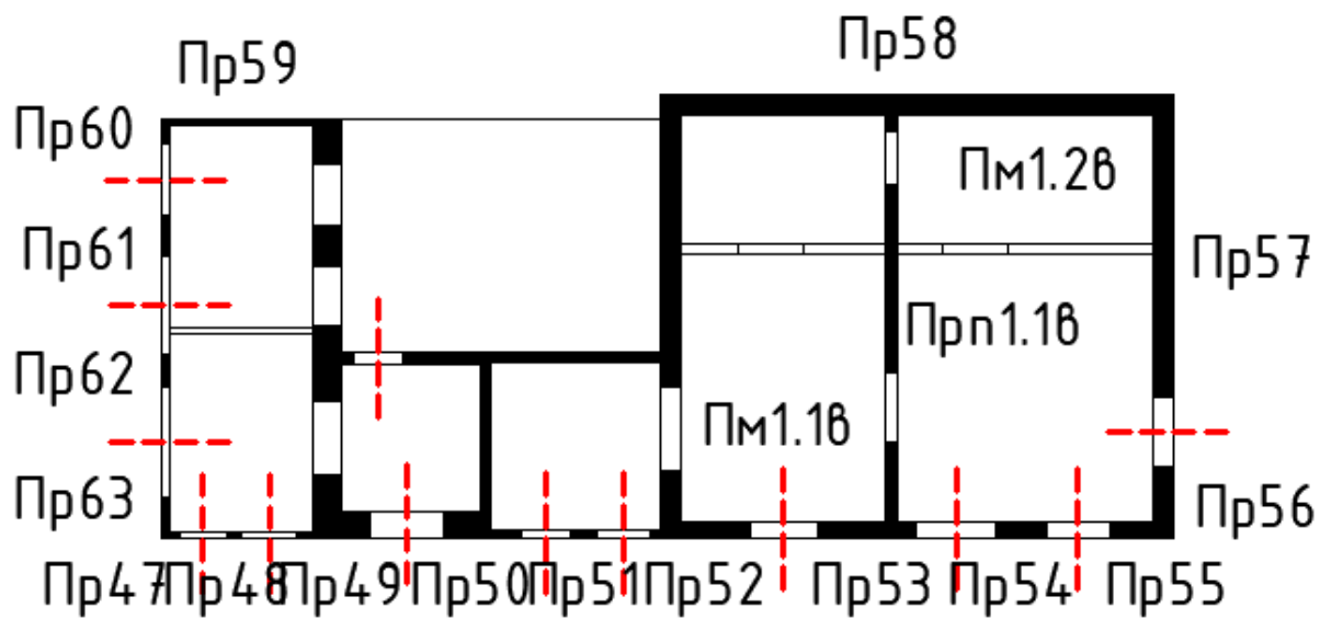
В-Фасад 1 (фундамент 1, стена 1, покрытие 1)
