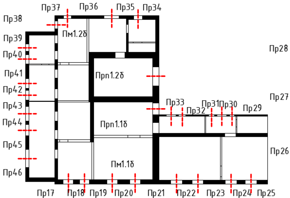
Б-План 1-ого этажа
