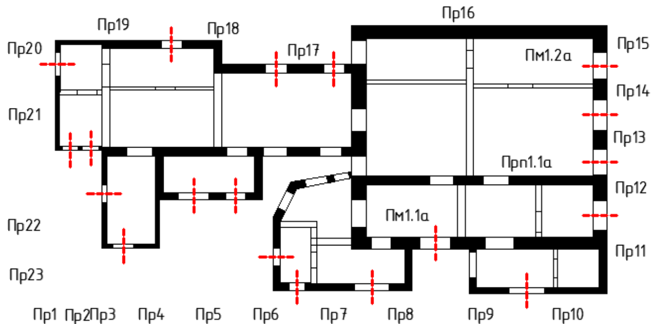
А-Фасад 1 (фундамент 1, стена 1, покрытие 1)
