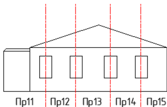
А-Фасад 3 (фундамент 3, стека 3, покрытие 3)
