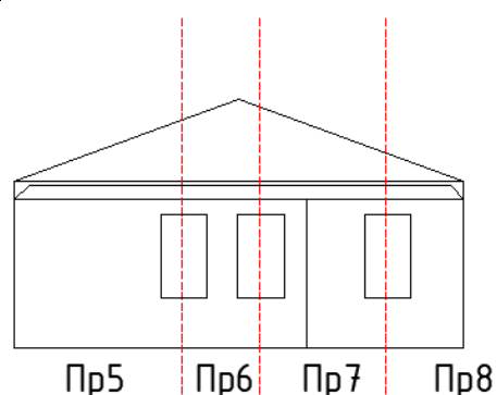
А-Фасад 4 (фундамент 4, стека 4, покрытие 4)
