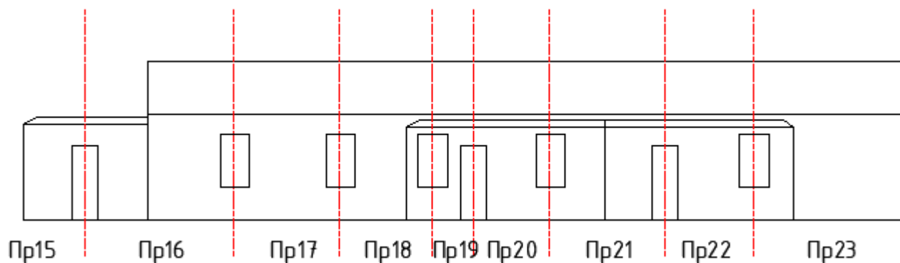
Б-Фасад 2 (фундамент 2, стена 2, покрытие 2)
