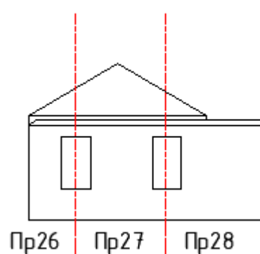
Б-Фасад 3 (фундамент 3, стена 3, покрытие 3)
