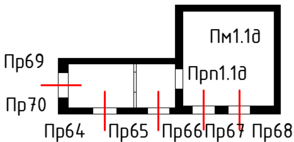
Д-Фасад 1 (фундамент 1, стена 1, покрытие 1)
