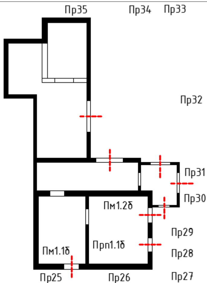
Б-Фасад 1 (фундамент 1, стена 1, покрытие 1)
