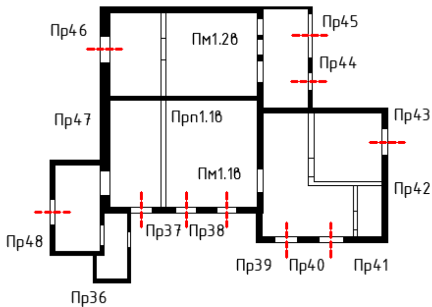
В-Фасад 1 (фундамент 1, стена 1, покрытие 1)
