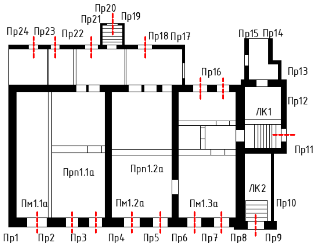
А-План 1-ого этажа
