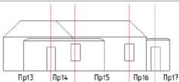
Б-Фасад 1 (фундамент 1, стена 1, покрытие 1)
