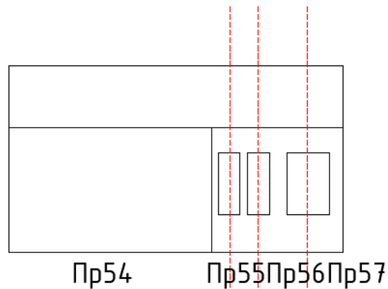
В-Фасад 2 (фундамент 2, стена 2, покрытие 2)
