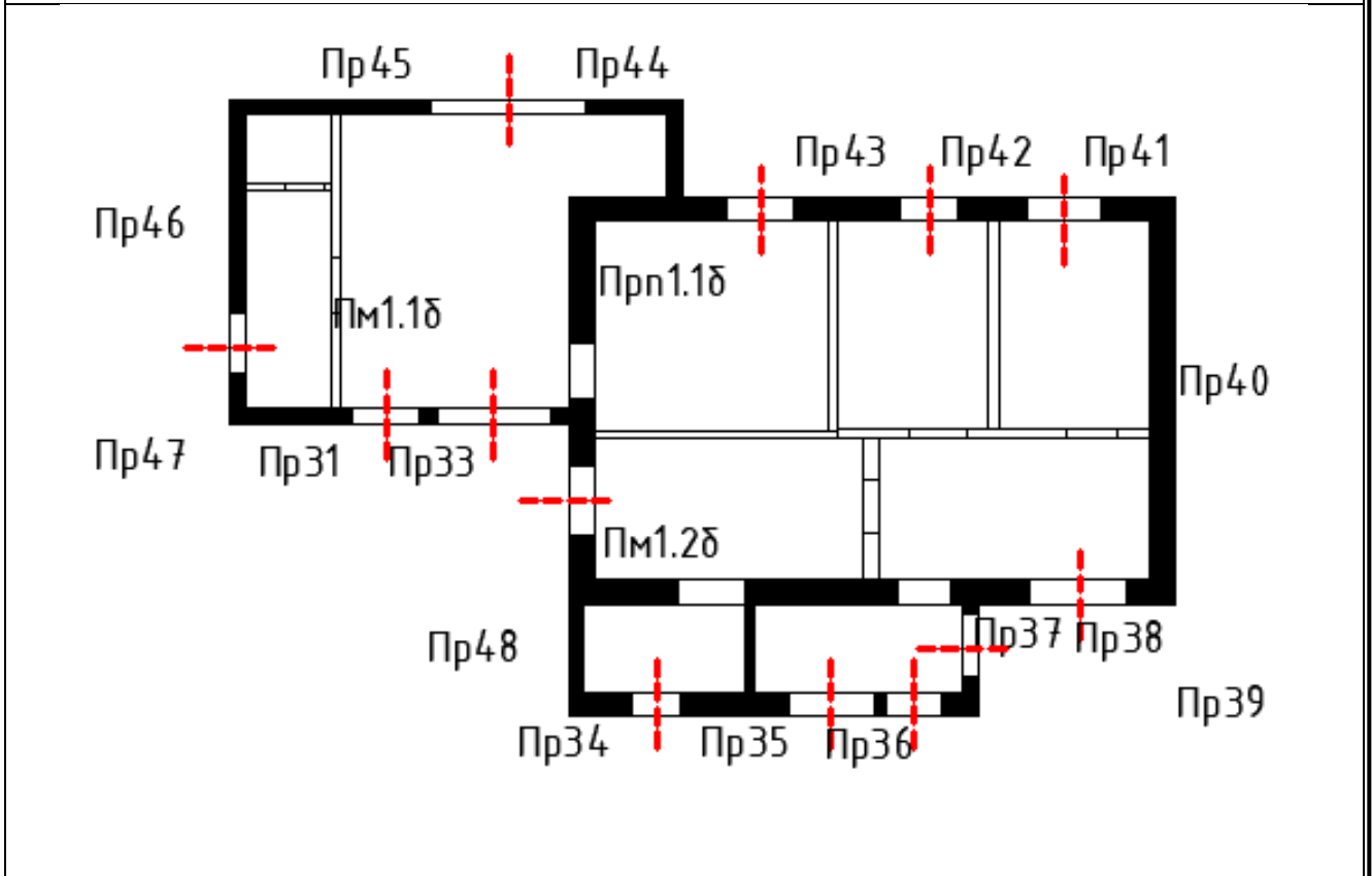
Б-План 1-ого этажа
