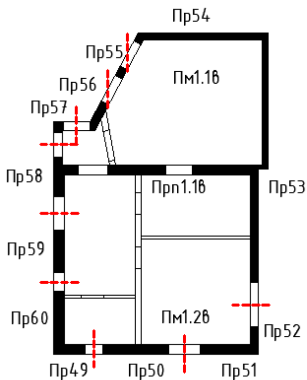
В-Фасад 1 (фундамент 1, стена 1, покрытие 1)
