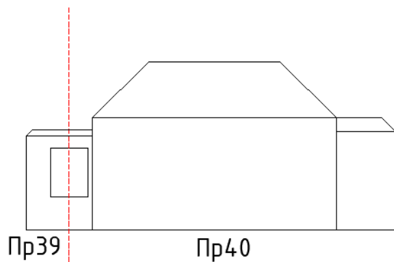
Б-Фасад 3 (фундамент 3, стена 3, покрытие 3)
