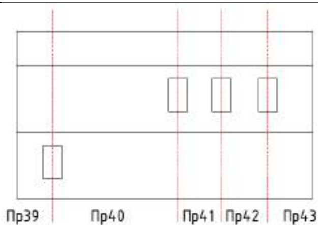
Б-Фасад 4 (фундамент 4, стена 4, покрытие 4)
