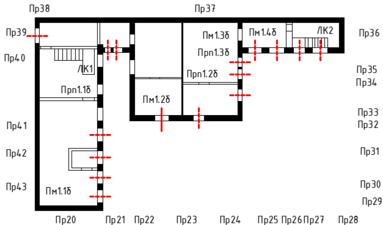
Б-План 2-ого этажа
