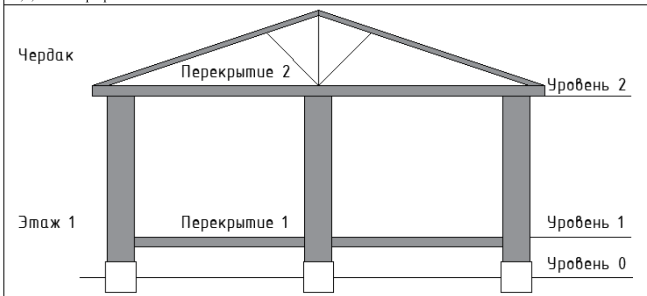
А,Б,В-Схема разреза
