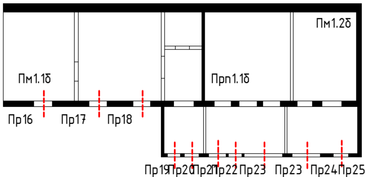
Б-Фасад 1 (фундамент 1, стена 1, покрытие 1)
