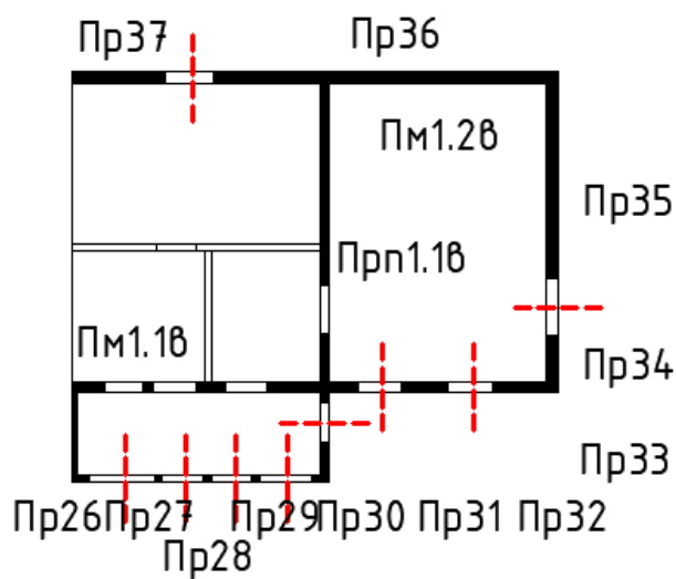
В-План 1-ого этажа
