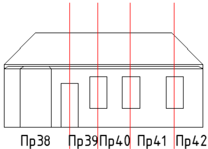
Б-Фасад 3 (фундамент 3, стена 3, покрытие 3)
