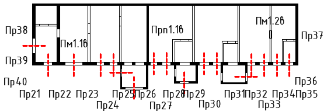
В-Фасад 1 (фундамент 1, стена 1, покрытие 1)
