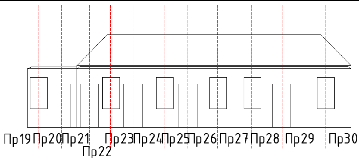
Г-Фасад 2 (фундамент 2, стена 2, покрытие 2)
